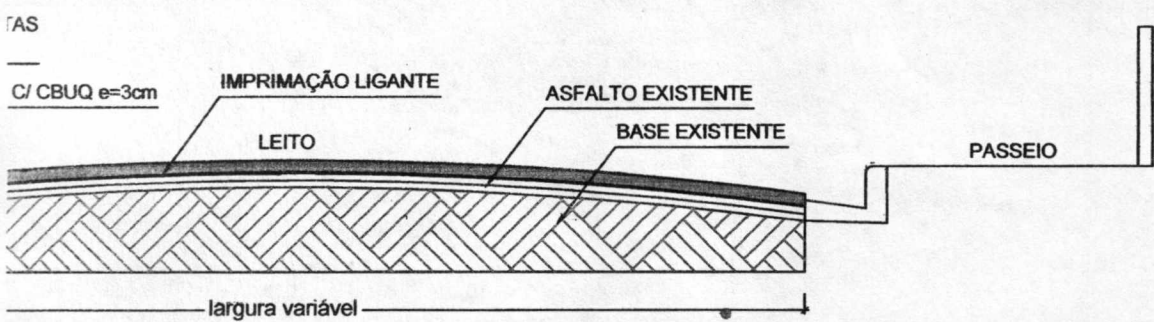
TE TRANSVERSAL ESQUEMÁTICO
