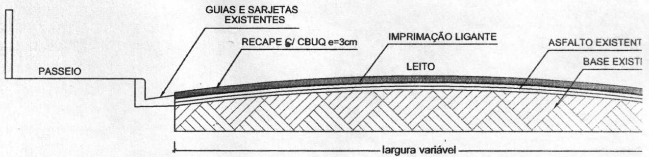
CORTE TRANSVERSAL ESQUEMÁTICO S/ESCALA
