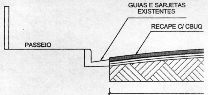
CORTE T S/ESCALA
