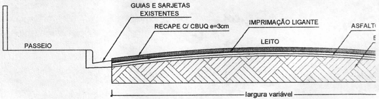
CORTE TRANSVERSAL ESQUEMÁTICO S/ESCALA
