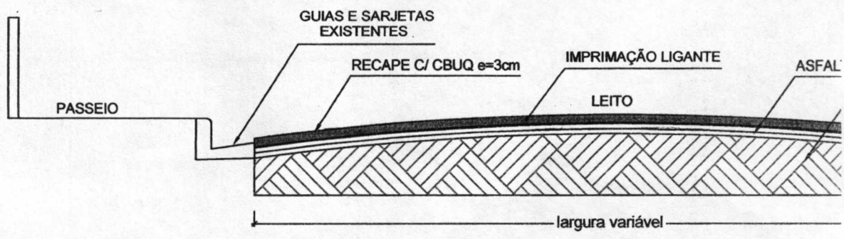
CORTE TRANSVERSAL ESQUEMA S/ESCALA
