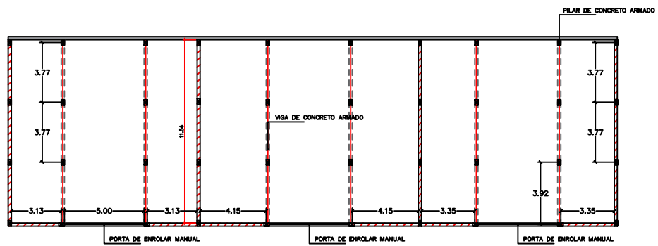
PLANTA BAIXA - VIGAS E PILARES Eac 1:100
